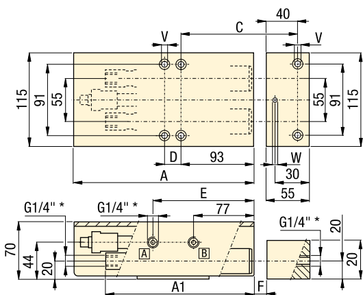
MCA-62, WCA-82 MPA-62
